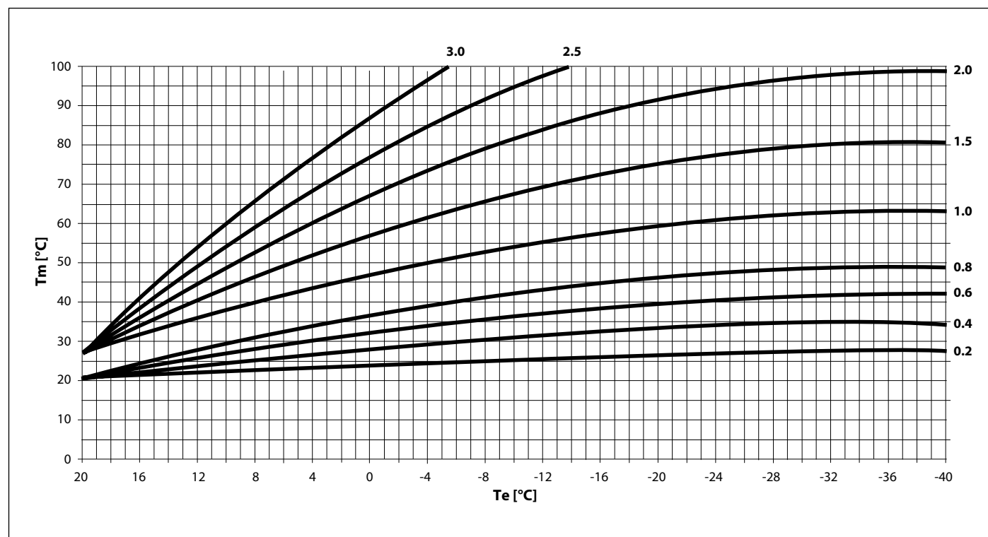
Obr. 24 Termoregulačné krivky
