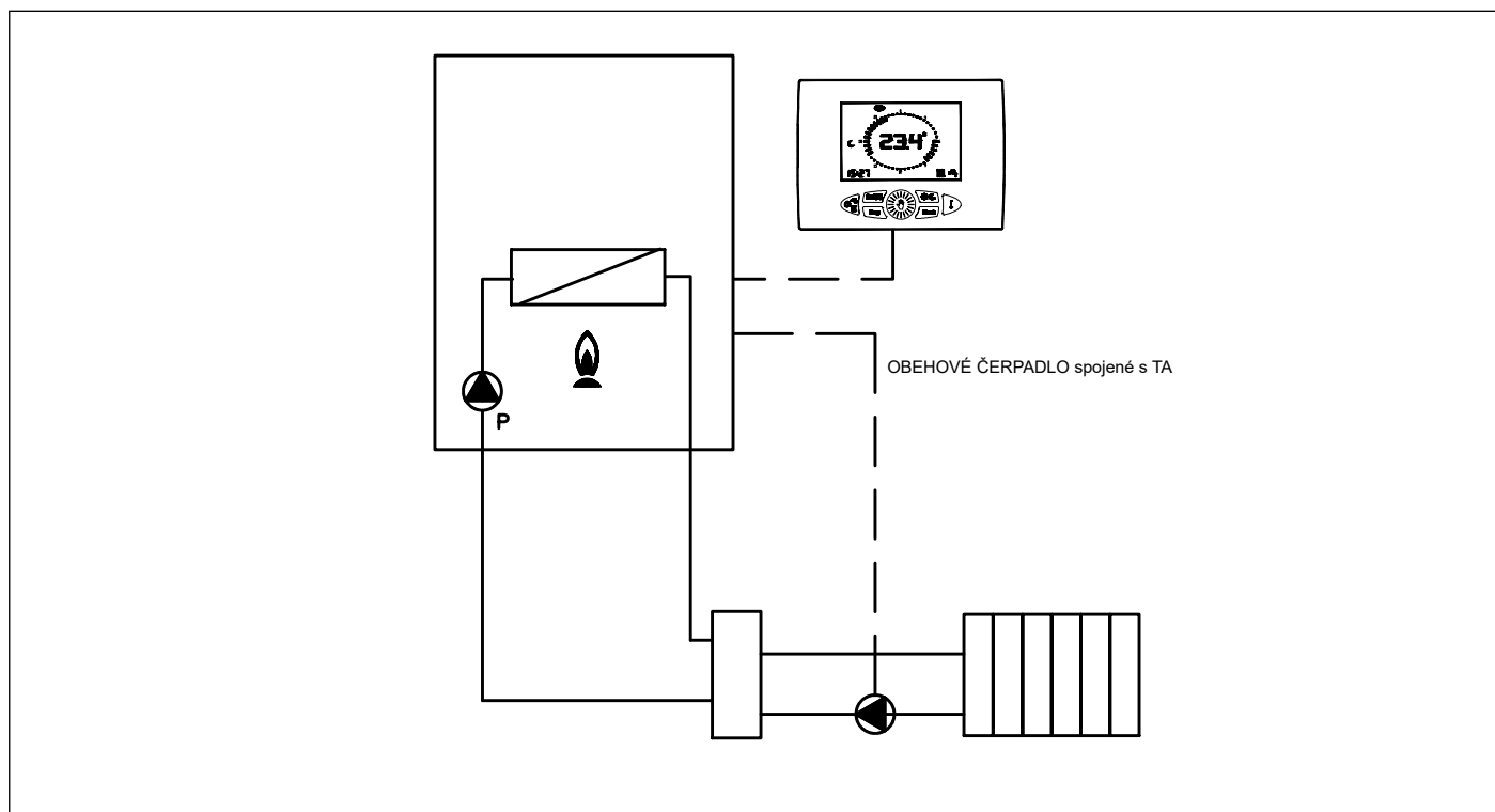
Obr. 29 Relé s diaľkovou požiadavkou (P17 = 1)
