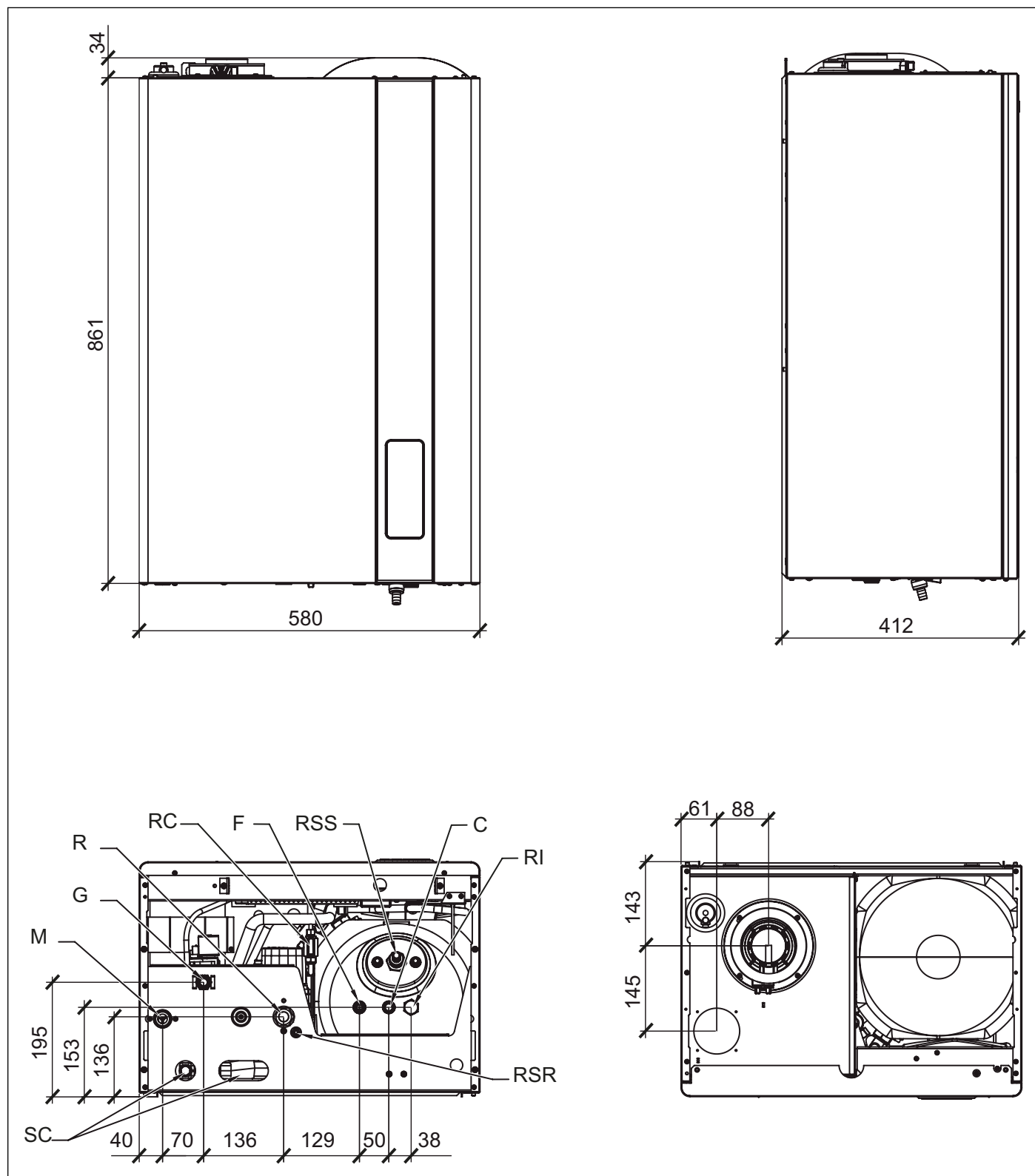
Obr. 3 Rozmery
