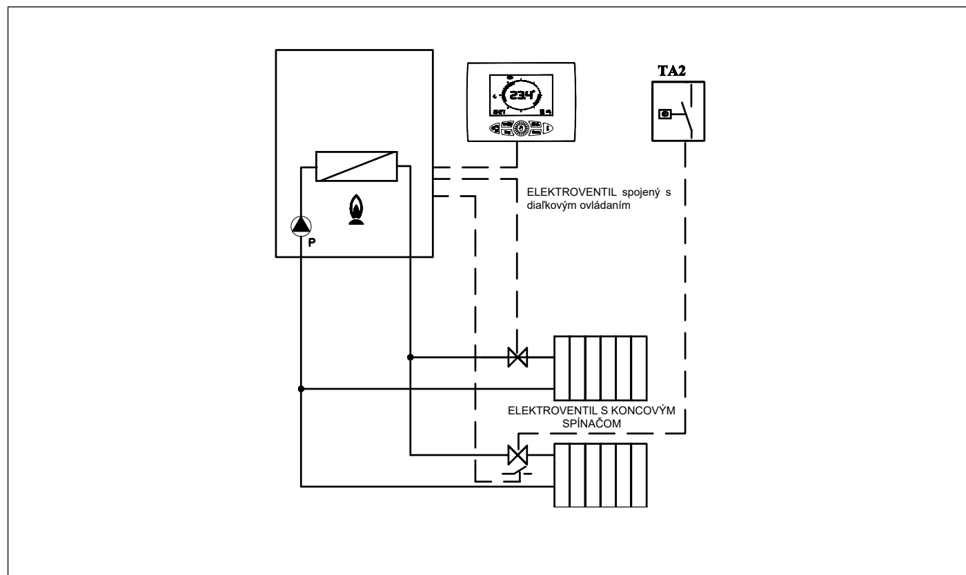
Obr. 27 Relé s diaľkovým ovládaním a TA2
