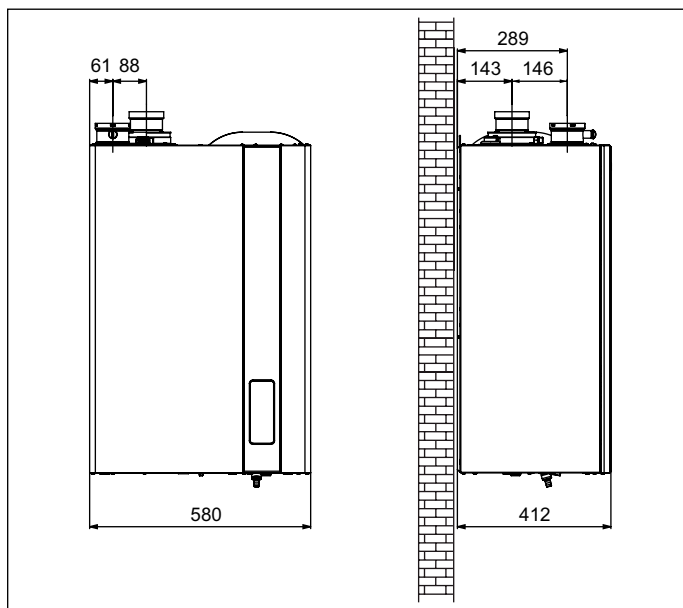
Obr. 18 Rozmery samostatných vedení typu C43 - C53 - C83
