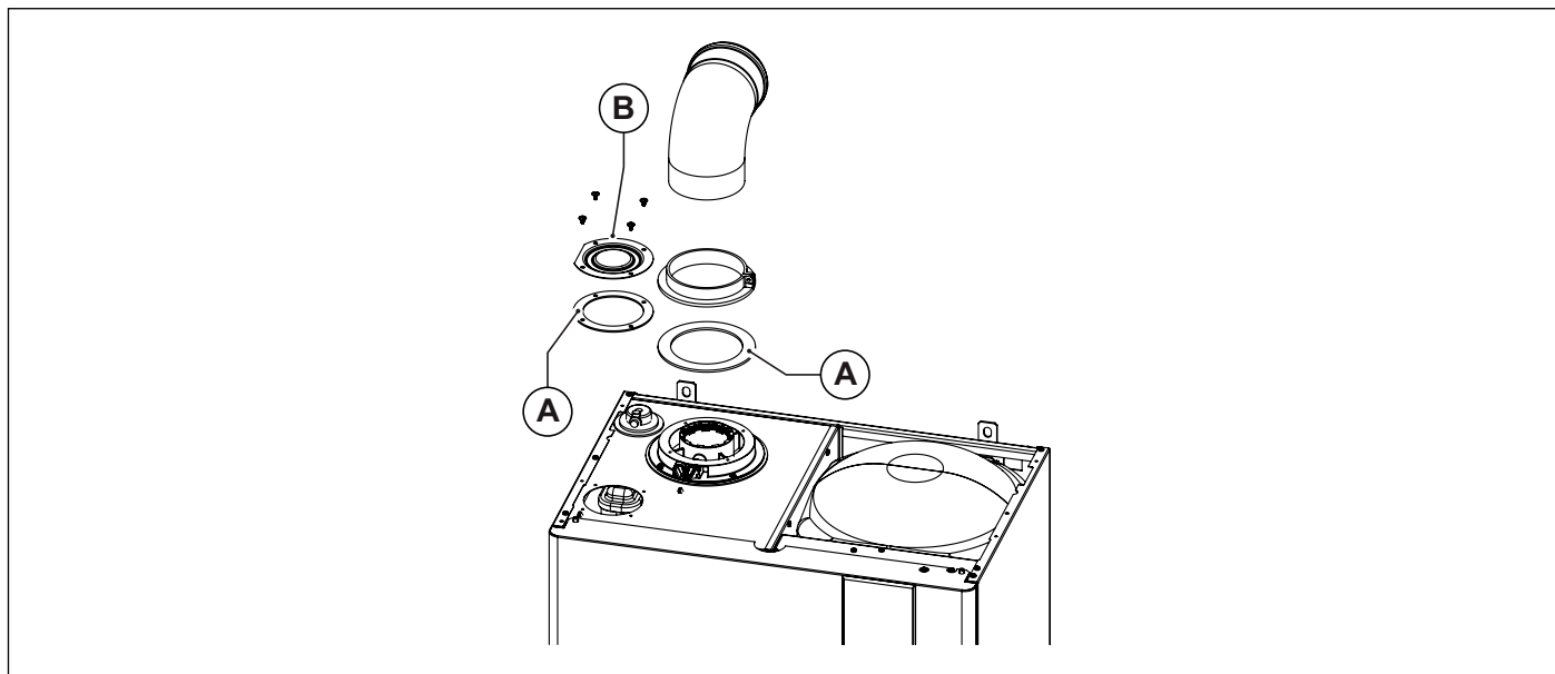
Obr. 15 Koaxiálne potrubia typu C13 - C33
