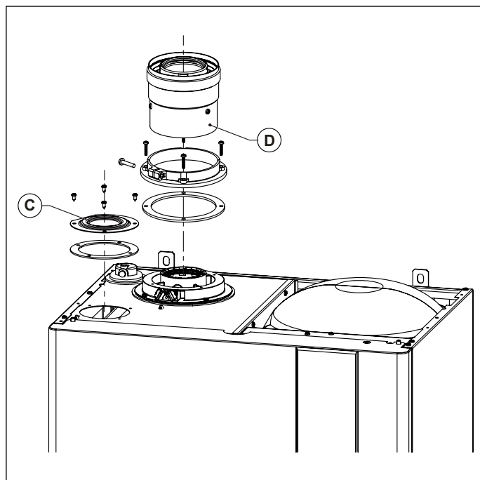
Obr. 9 Inštalácia koaxiálnej súpravy
