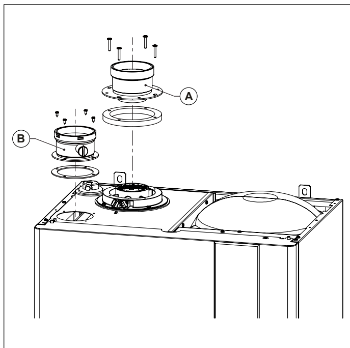
Obr. 8 Inštalácia súpravy s dvojitém potrubím
