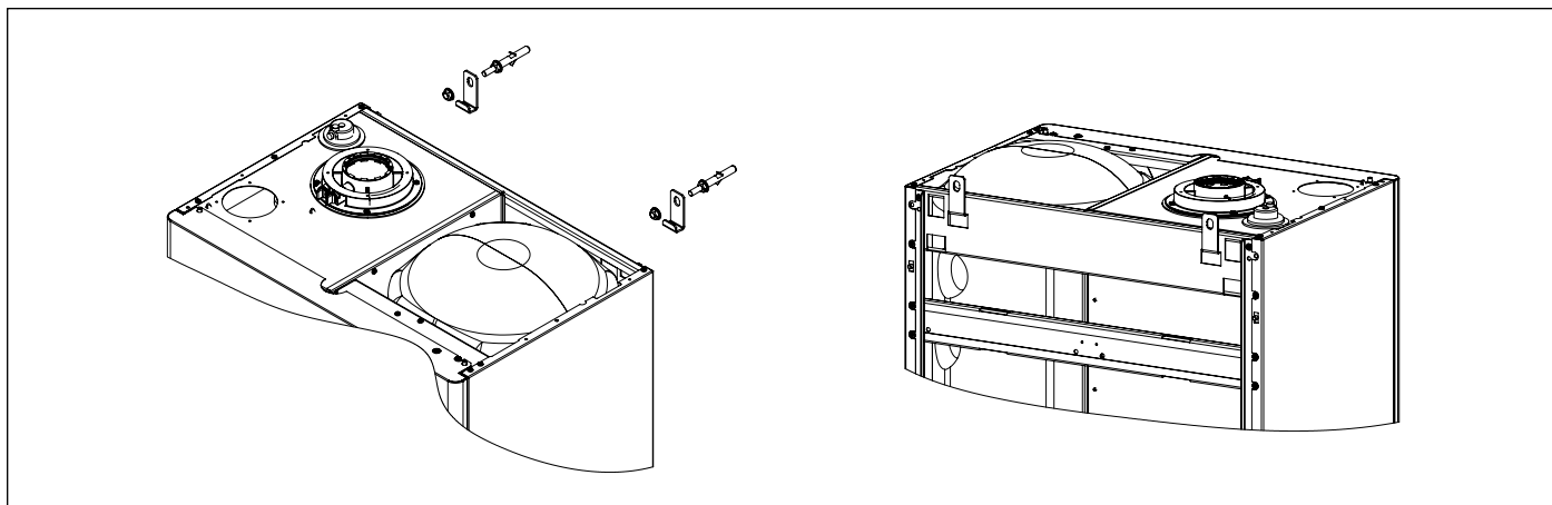
Obr. 7 Upevnenie konzol
