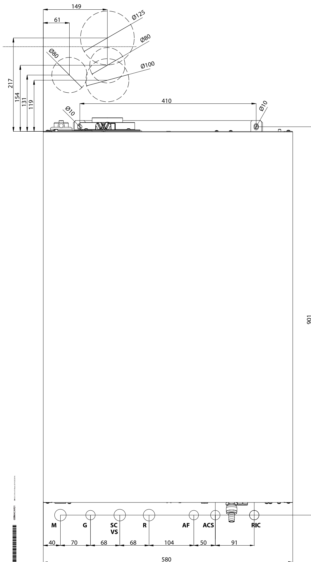
Obr. 6 Kartónová šablóna
