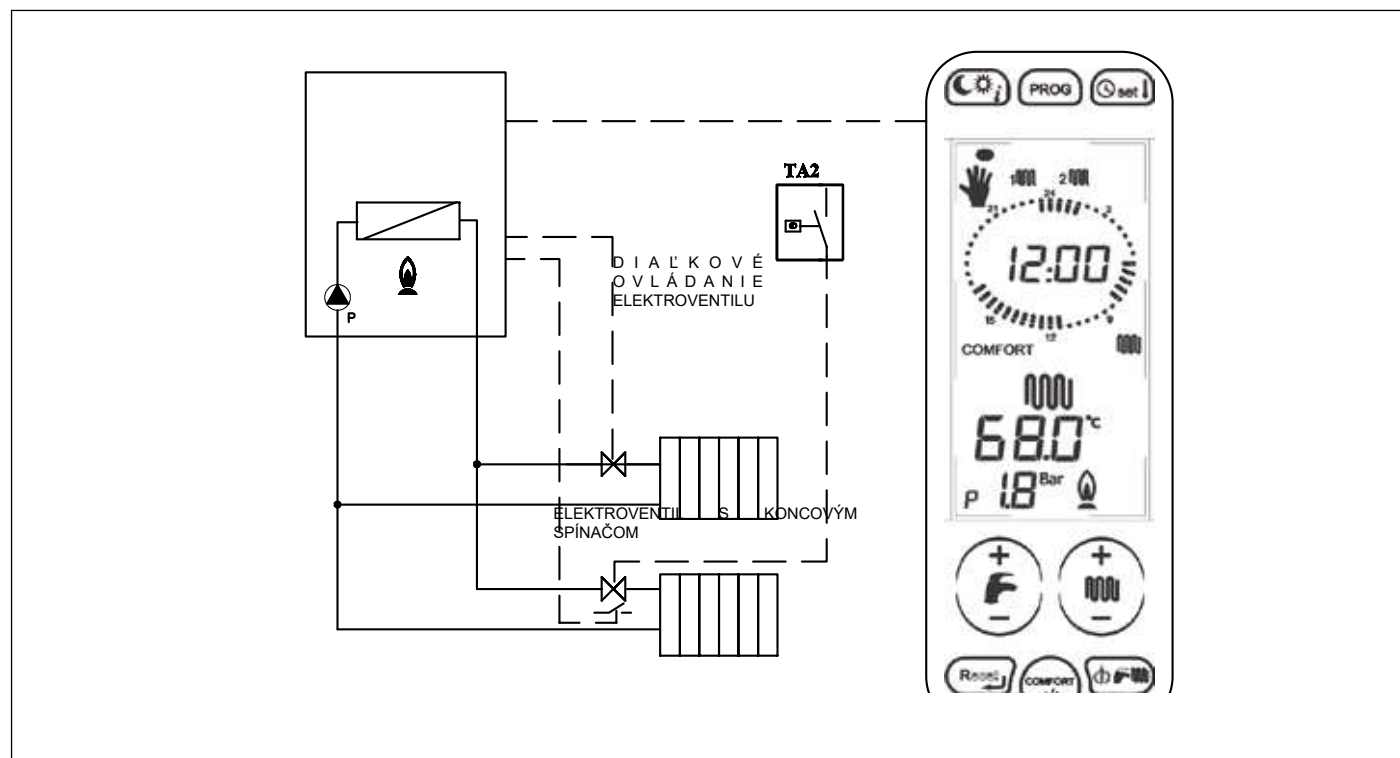
Obr. 28 Relé s programom rozhrania a TA2
