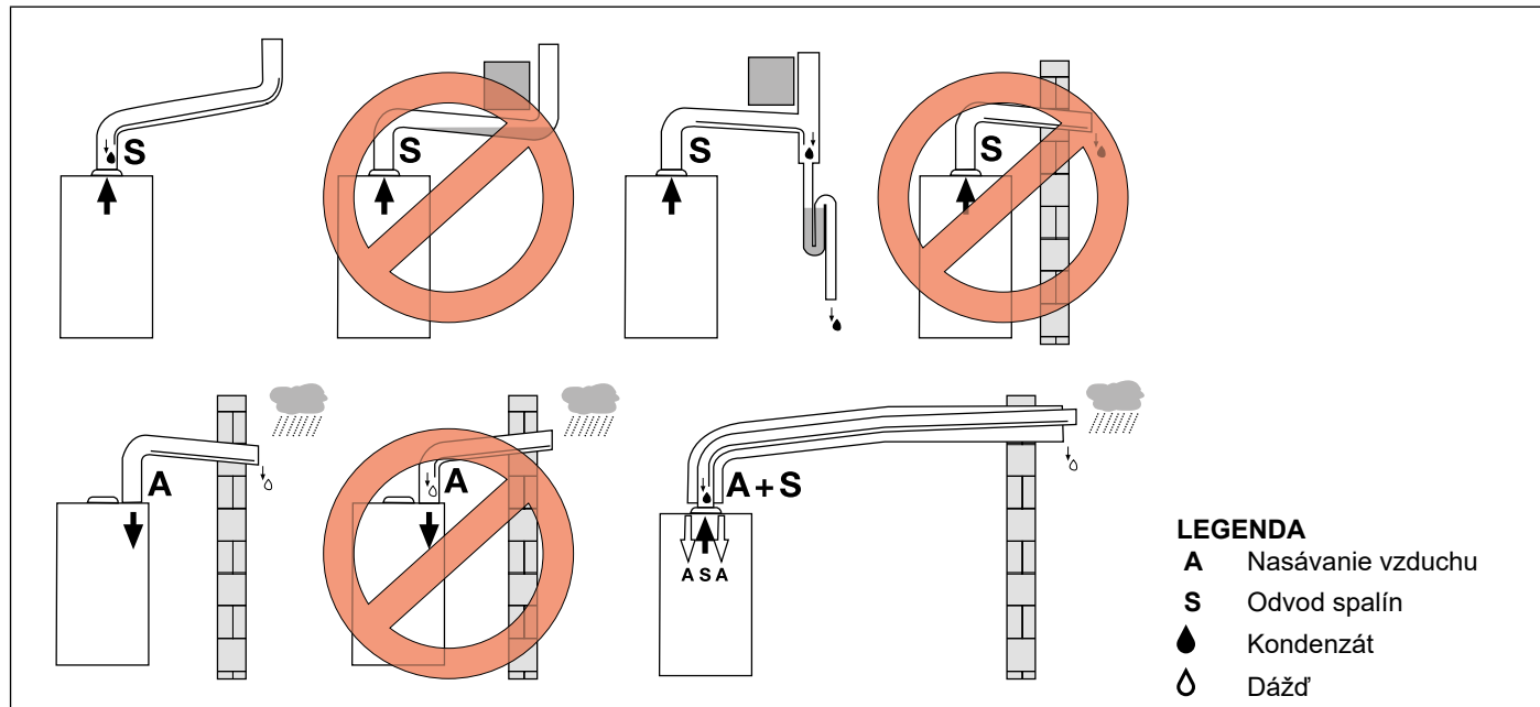
Obr. 10 Príklady inštalácie
