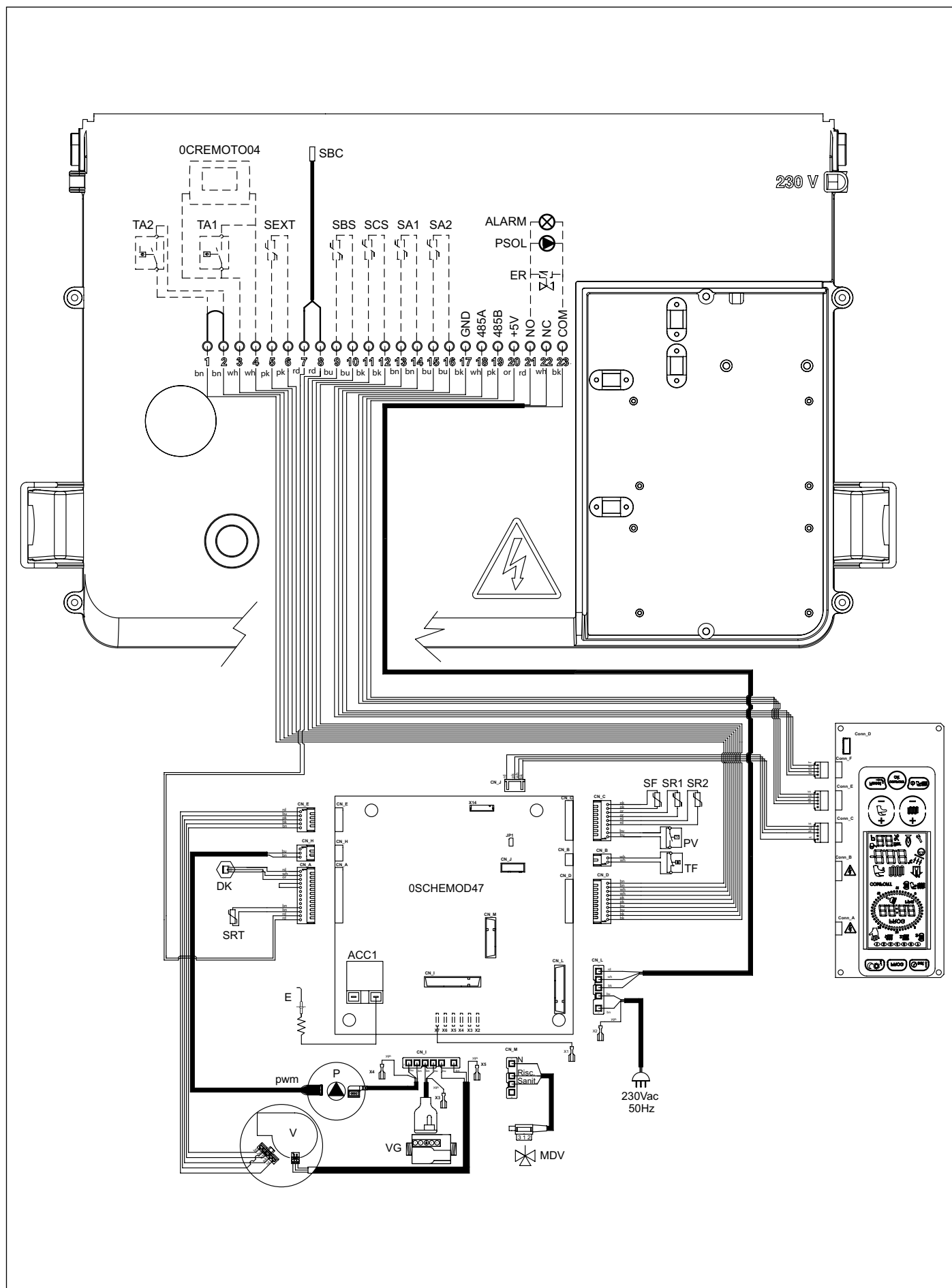
Obr. 25 Elektrická schéma
