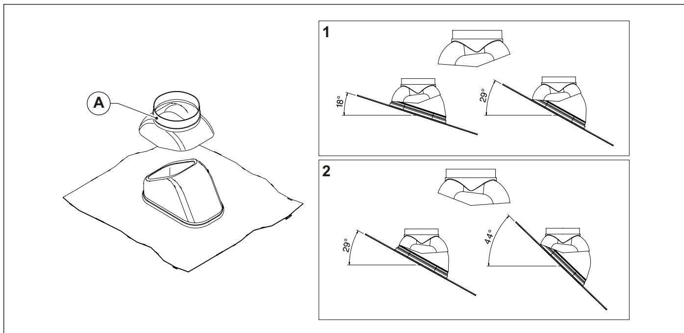
Obr. 13 Škridla pre naklonené strechy
