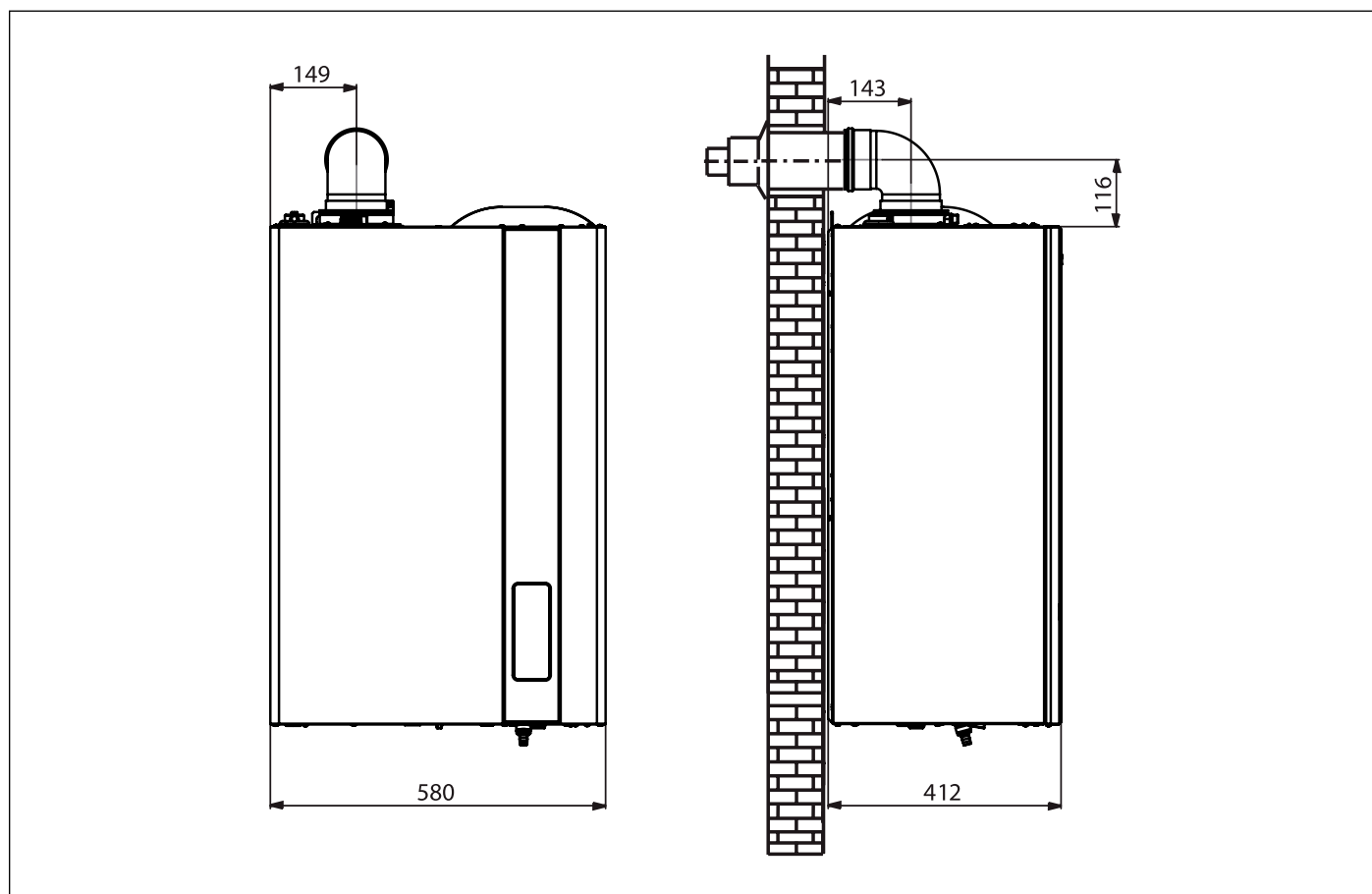
Obr. 16 Veľkosť koaxiálneho potrubia typu C13 - C33
