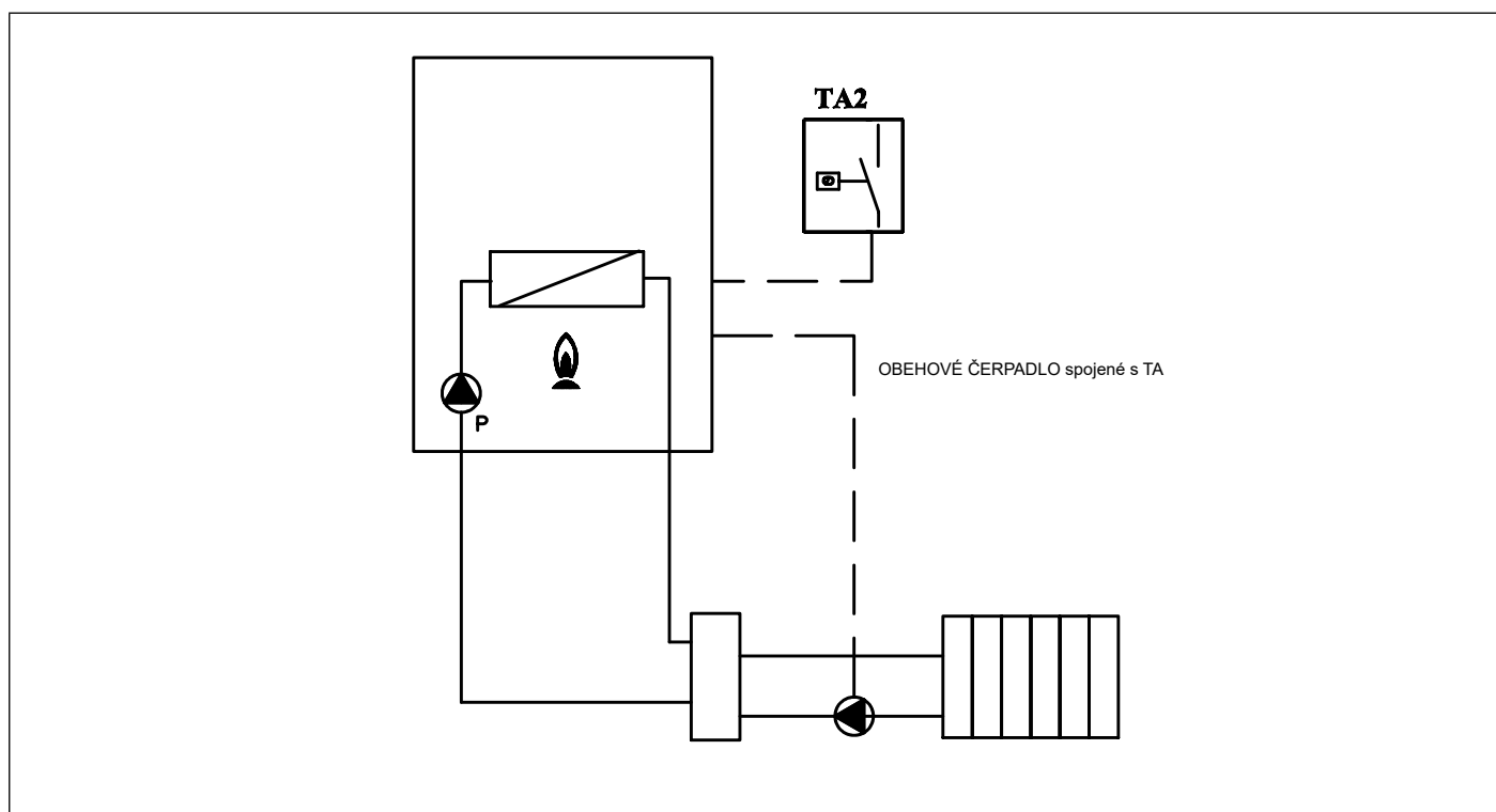
Obr. 30 Relé s požiadavkou (P17 = 3)
