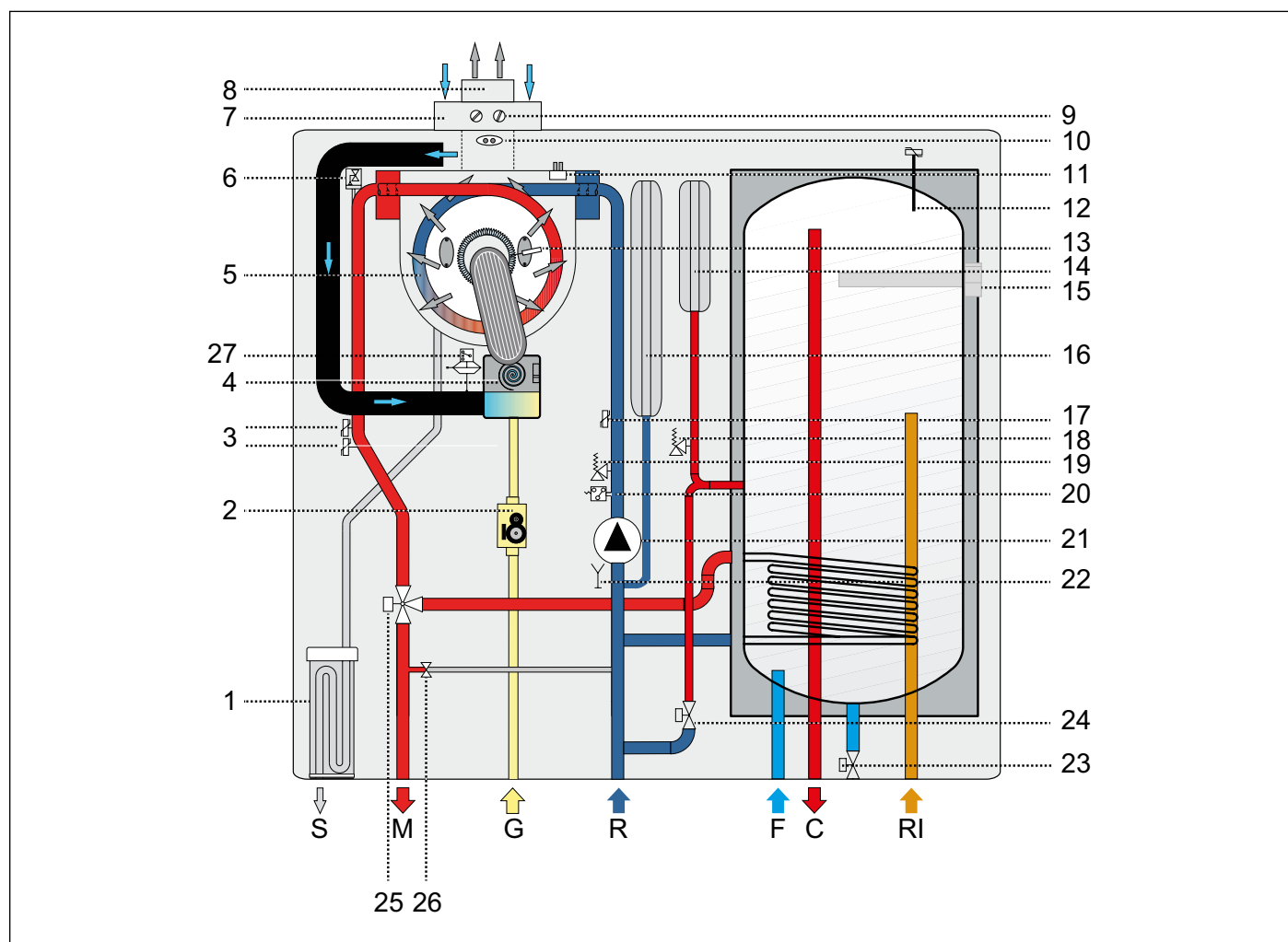
Obr. 5 Hydraulická schéma
