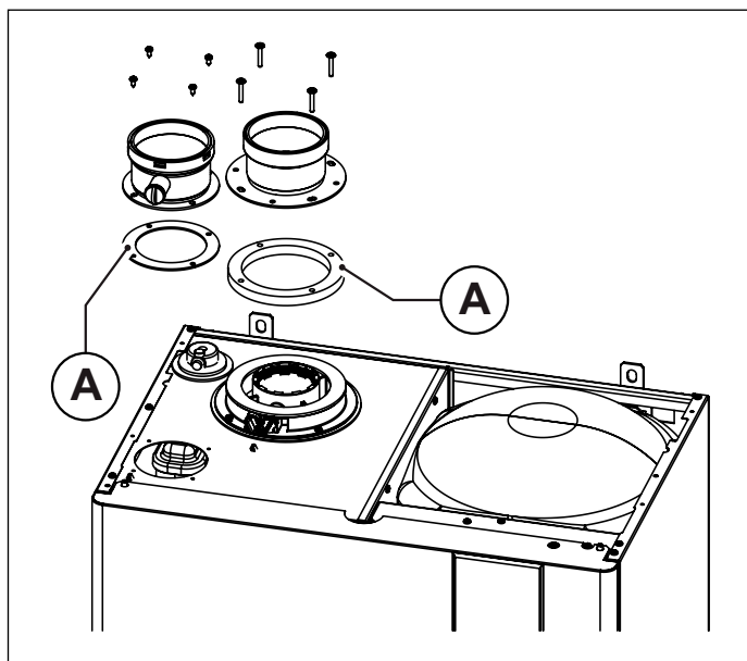
Obr. 17 Samostatné vedenia typu C43 - C53 - C83
