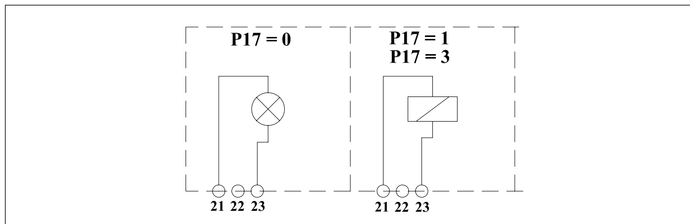
Obr. 26 Schéma zapojenia multifunkčného relé
