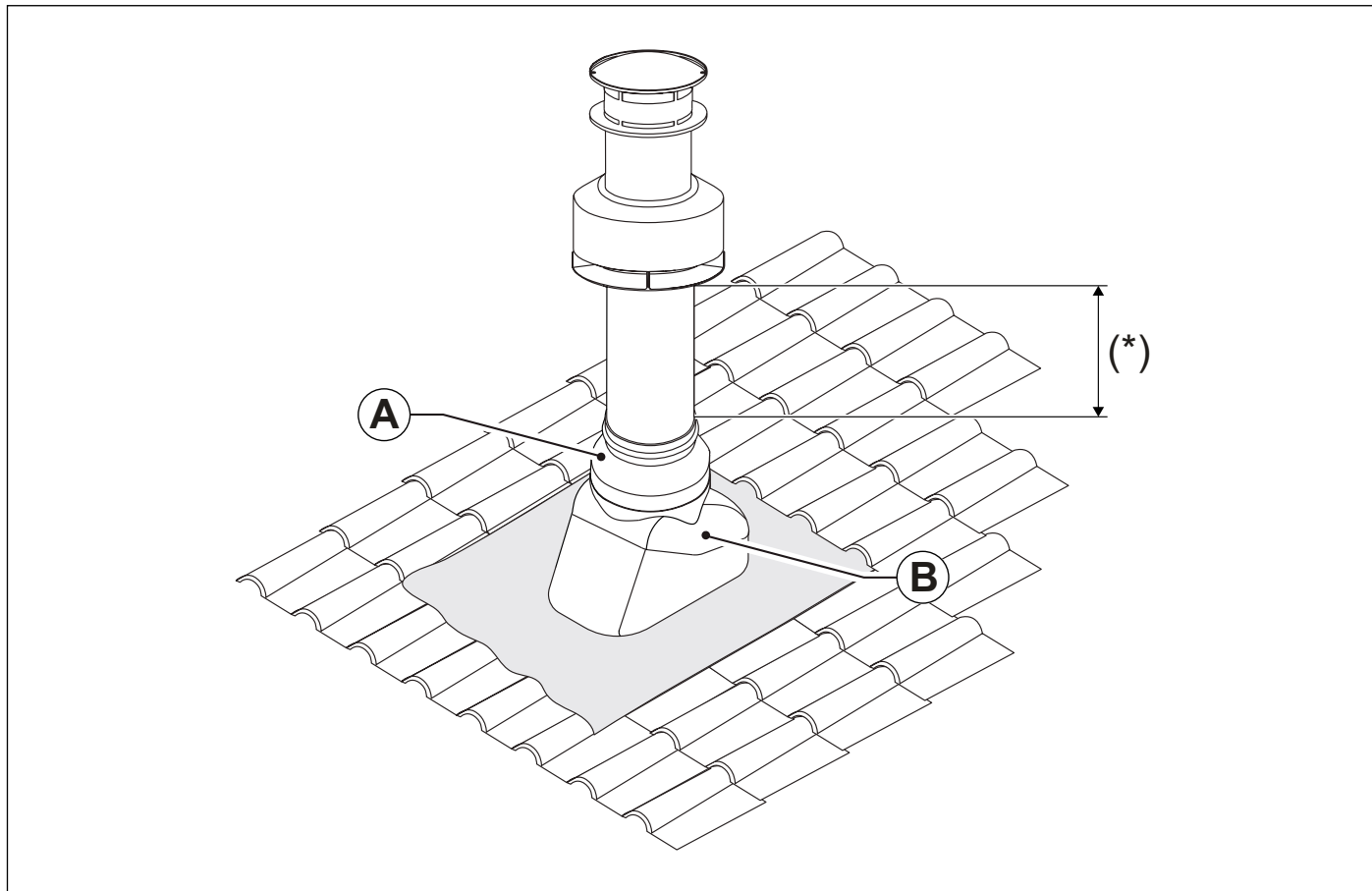
Obr. 14 Inštalácia dymovodu so strieškou
