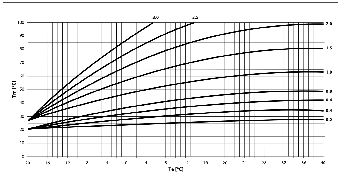
Obr. 22 Termoregulačné krivky
