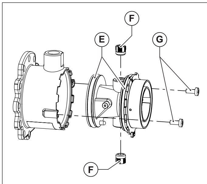
Obr. 34 Plastové teleso zmiešavača
