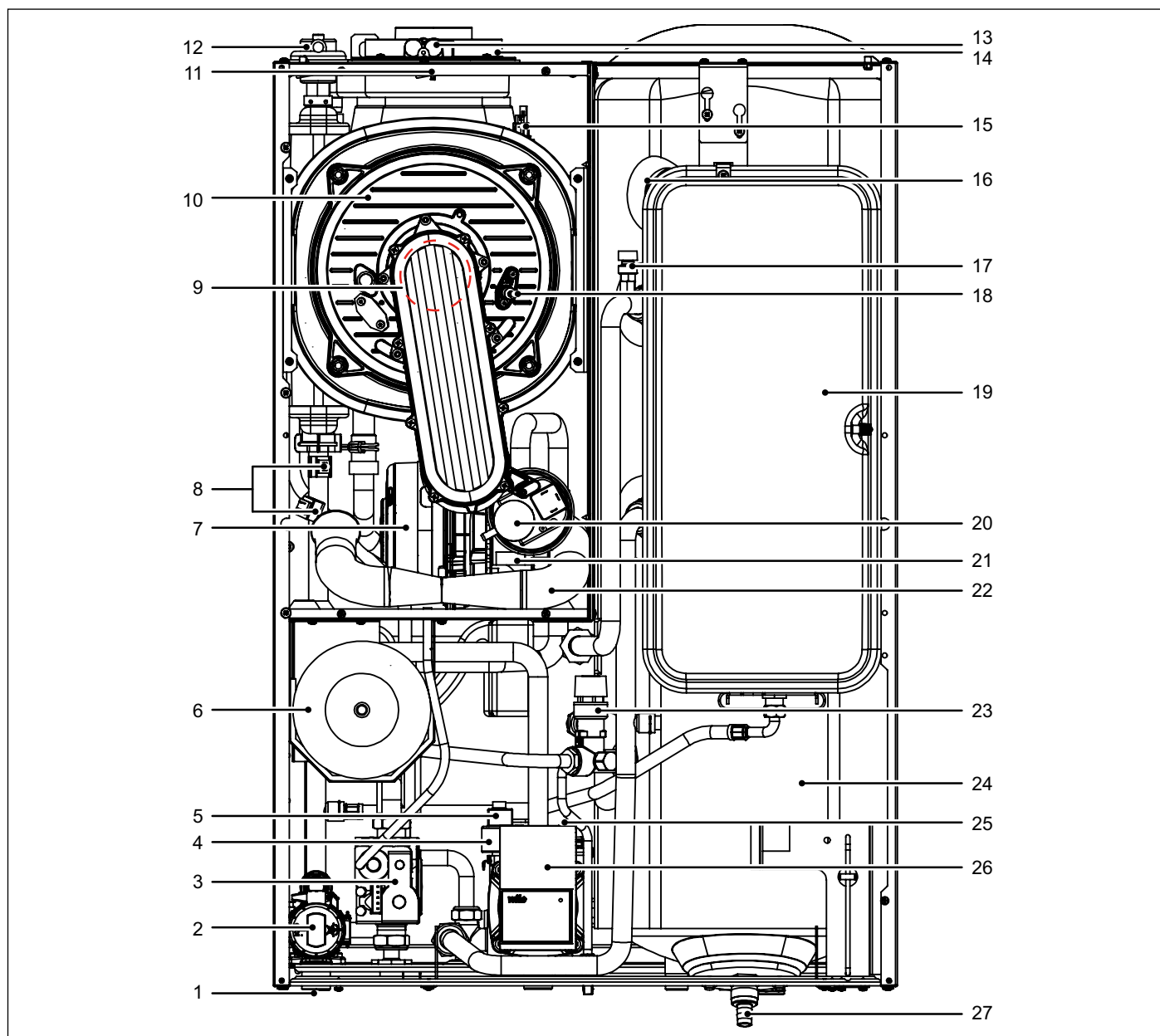
Obr. 4 Hlavné súčasti
