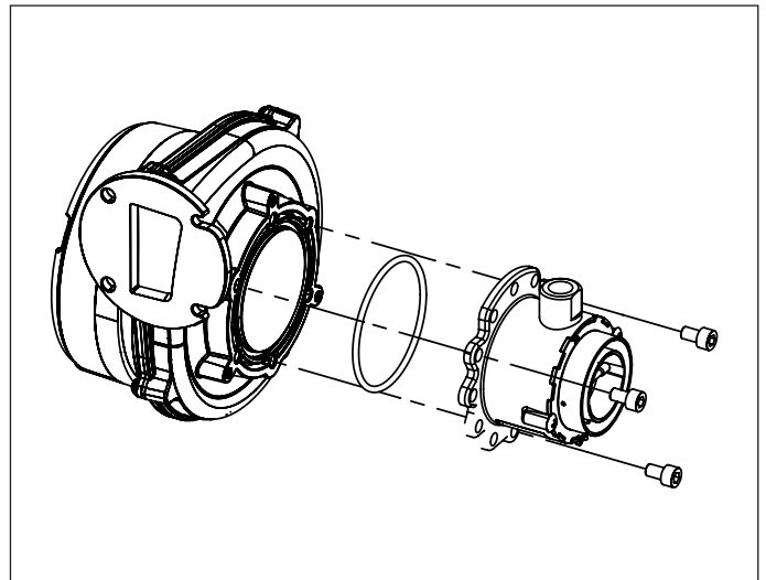
Obr. 31 Zmiešavač
