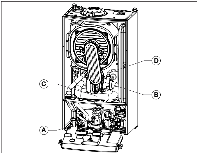
Obr. 30 Tlmič nasávania
