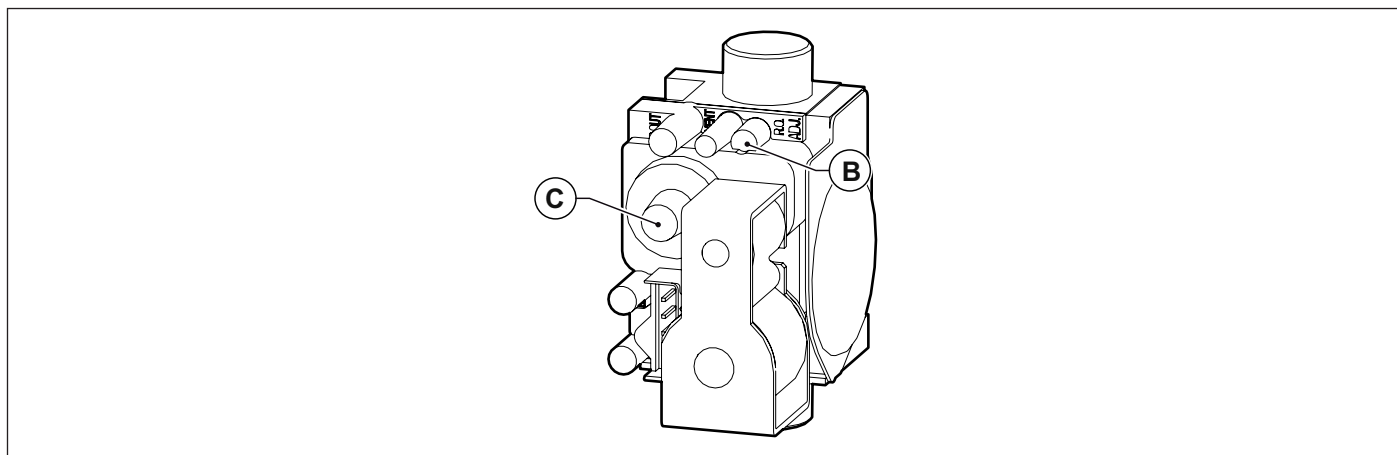
Obr. 34 Regulácia hodnoty oxidu uhličitého
